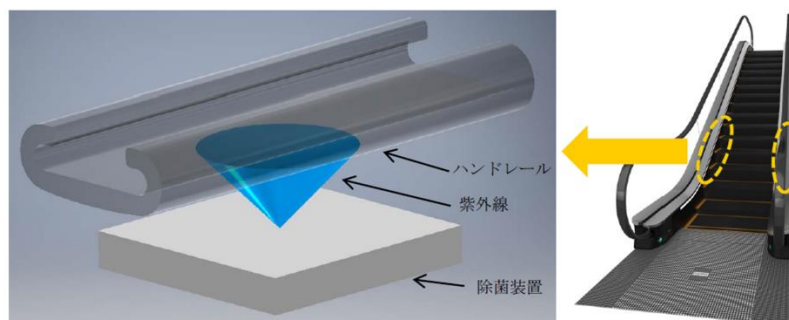
ハンドレール除菌装置の構造図（イメージ）
